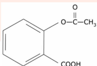
Fórmula estructural.
